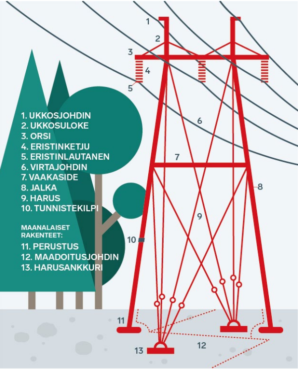
Kuva 2. Voimajohdon rakenneosat
