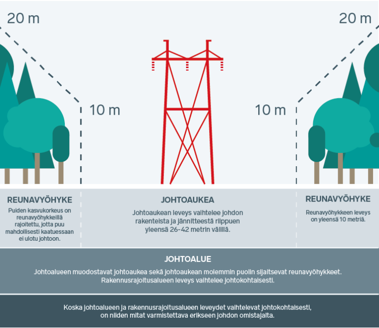
Kuva 1. Johtoalueen kaaviokuva
