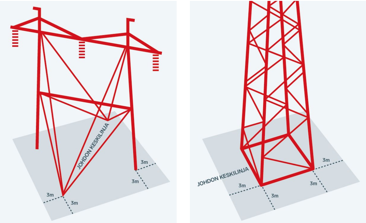
Kuva 3. Harustetun ja vapaasti seisovan pylvään pylväsalan kaaviokuva
